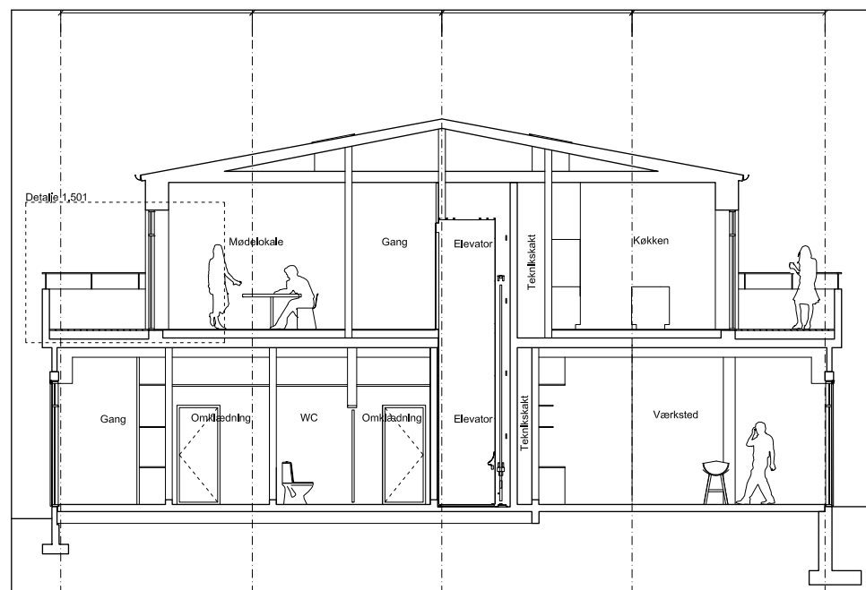
Sektion genom klubbhuset visar exempelvis en liten hiss som ökar tillgängligheten.
