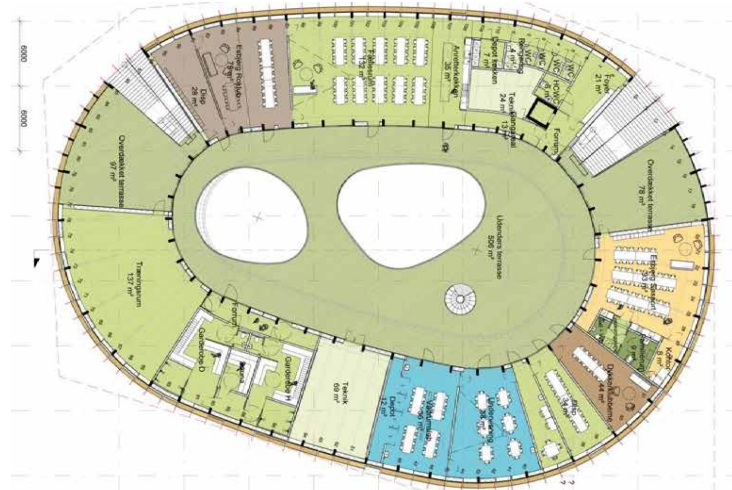
Planritning övre plan. Grön färg är offentliga eller delade utrymmen.
